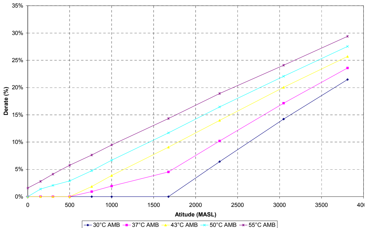
Derate Chart 2206C-E13 TAG2 400 kVA Low E
