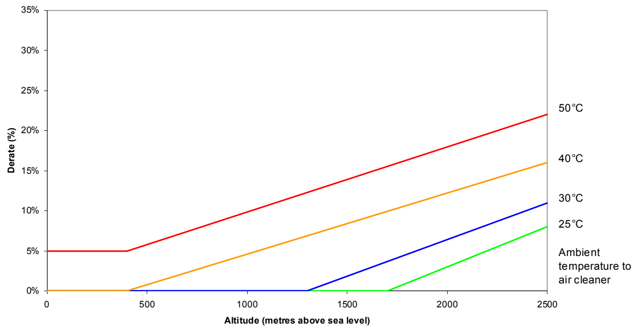
4008TAG1A 1500rpm Altitude/Ambient Derate
